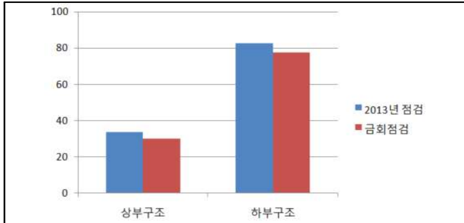
【그림 4.4】 부재별 탄산화깊이에 의한 콘크리트 잔여피복두께 비교
